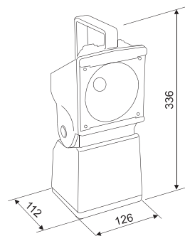
Bild3:Abmessungen HaloLux90ALED Typ4540...
